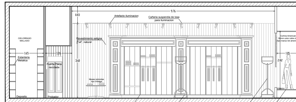
CORTE A-A
