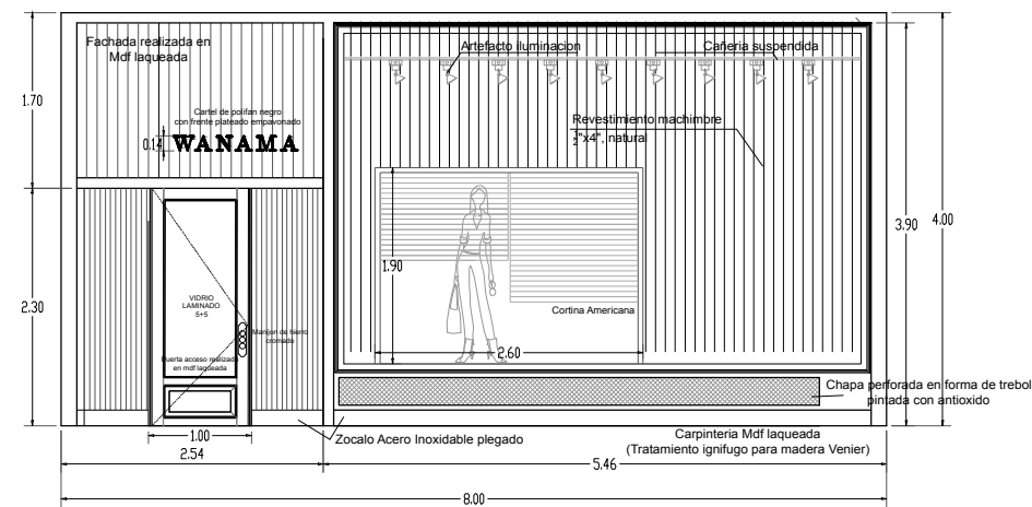
FACHADA
