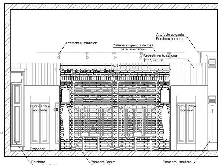
CORTE C-C
